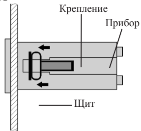
Рис. 2 – Установка прибора
